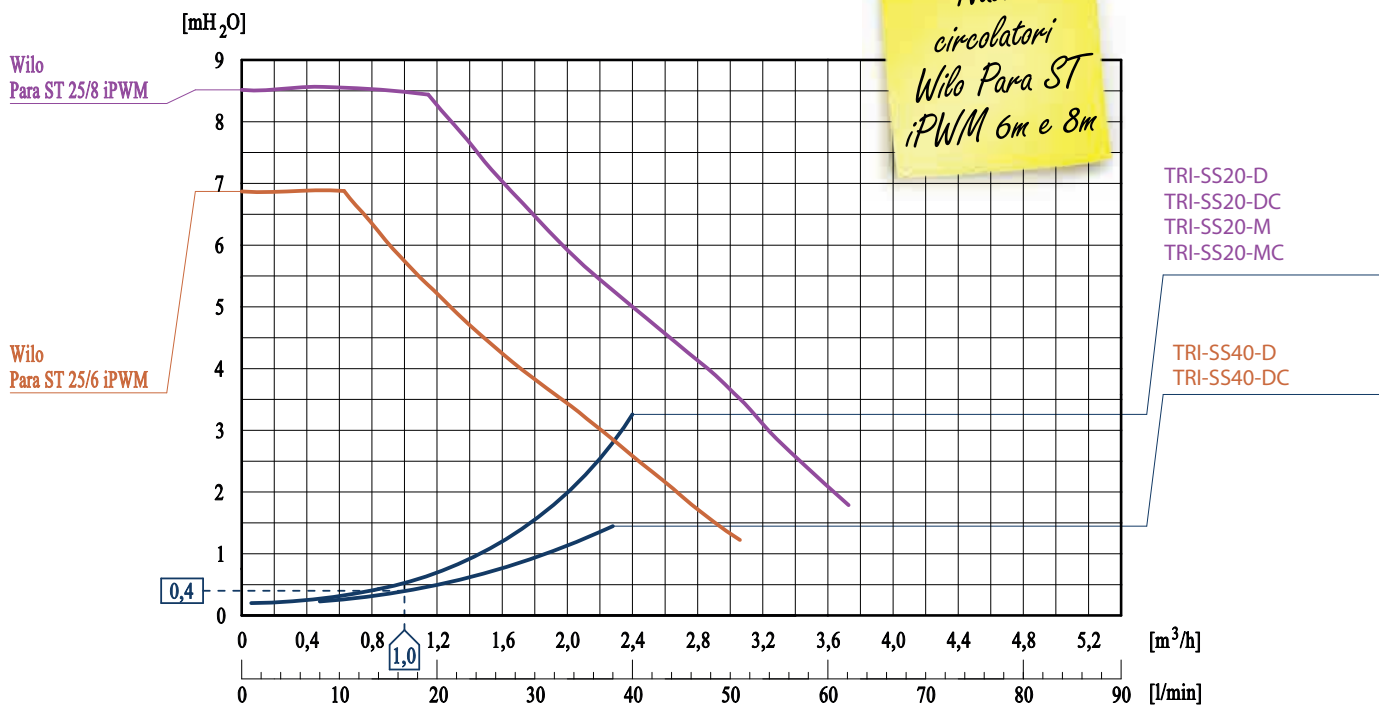
Curve caratteristiche dei moduli e dei circolatori
