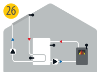
26 Solare con accumulo e caldaia a legna
