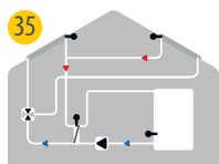
35 2x Solare con accumulo, scambiatore e valvola
