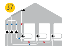
37 Solare con 3 accumuli e 3 pompe
