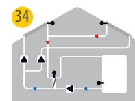
34 2x Solare con accumulo, scambiatore e 3 pompe
