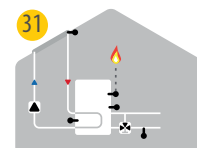
31 Solare con termostato e innalzamento ritorno
