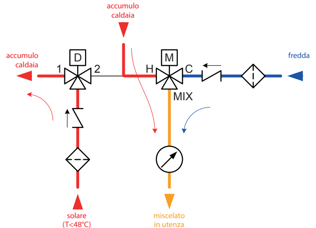
Schema 2: funzionamento con una temperatura dell'accumulo solare inferiore a 48°C
