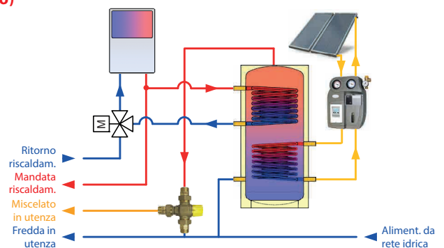
Circolazione forzata (impianto glicole / circuito chiuso) ed integrazione con caldaia
