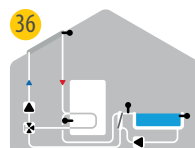
36 Solare con piscina, accumulo, scambiatore e valvola
